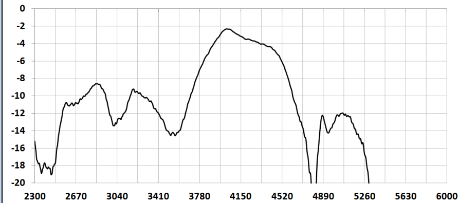
Rückflußdämpfung / Return loss
