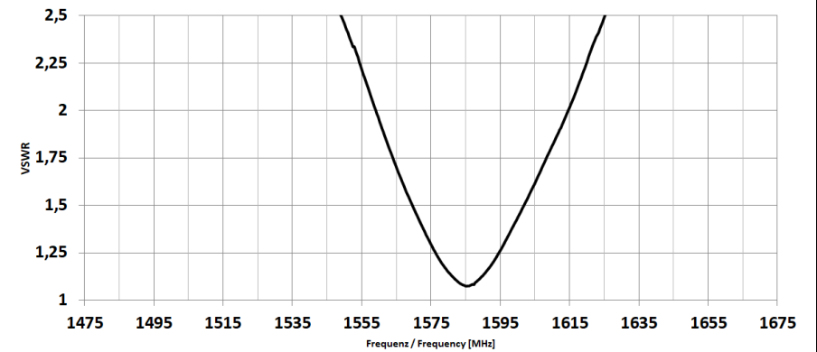
VSWR
