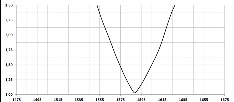
VSWR
