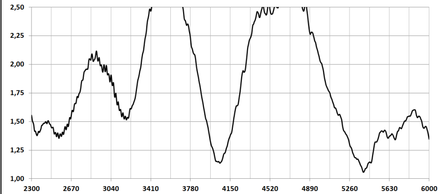
VSWR
