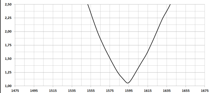
VSWR
