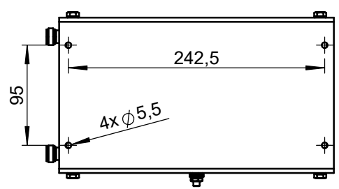
Ansicht von unten / Befestigungsmaße
