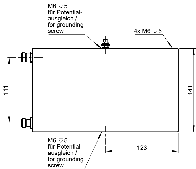
Ansicht von unten / Befestigungsmaße
